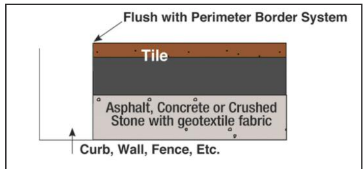
Flush Tile Edge
